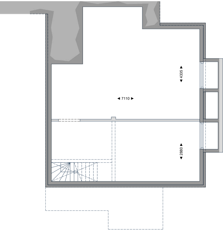
Kelder
