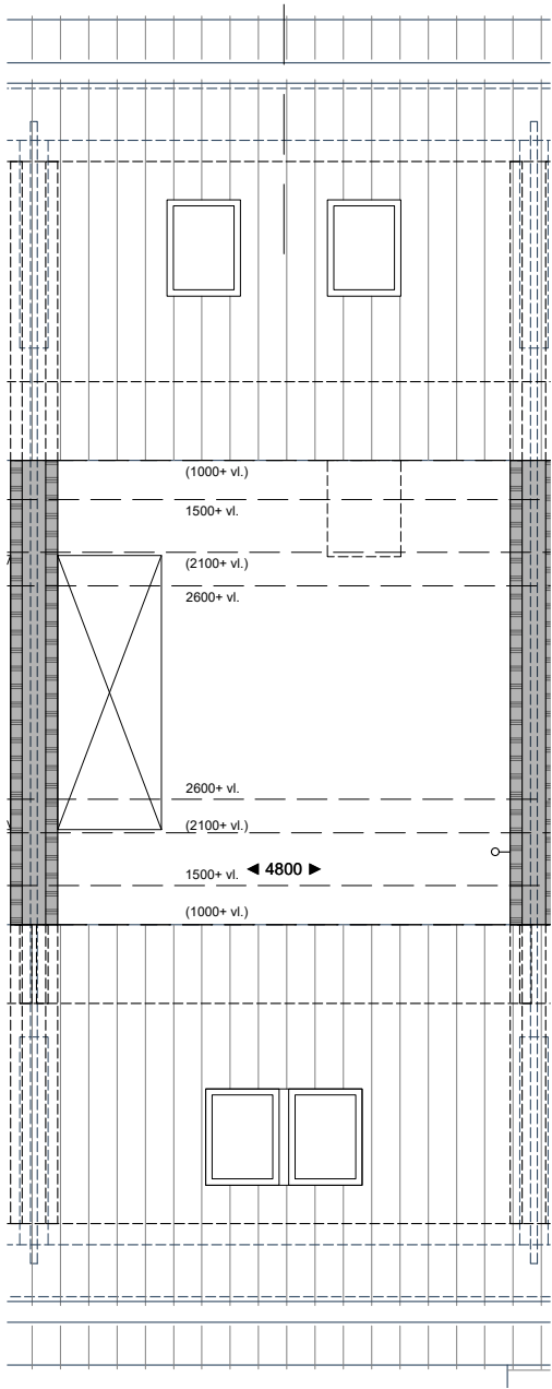
Derde verdieping
