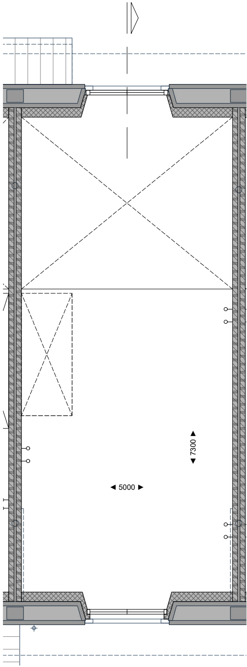
Eerste verdieping
