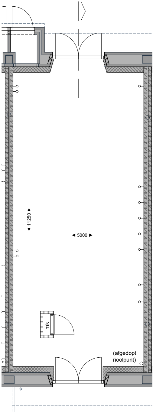
Begane grond
