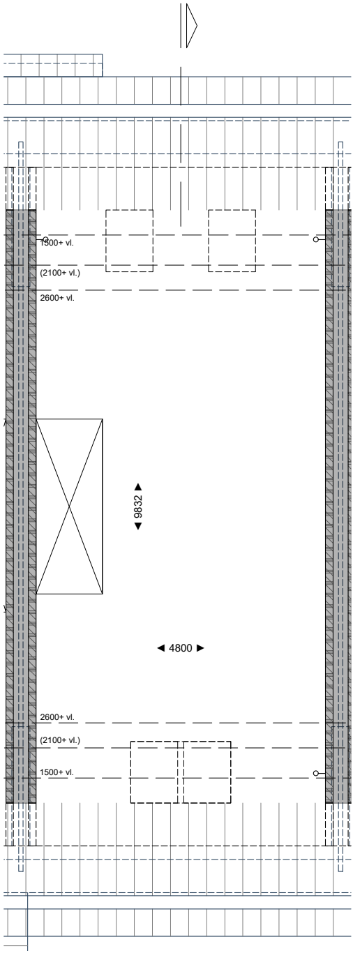
Tweede verdieping
