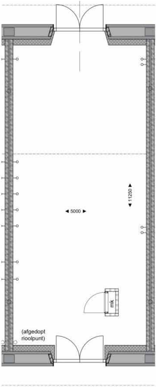
Begane grond
