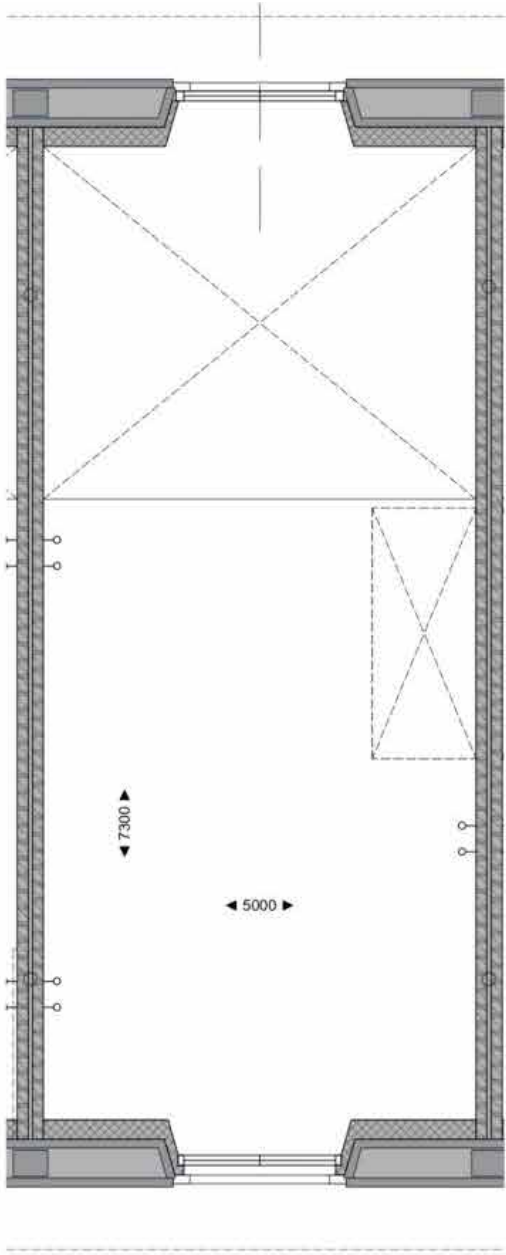
Eerste verdieping
