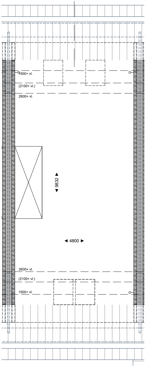
Tweede verdieping
