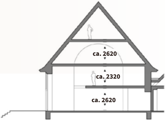
Principedoorsnede (1) woning 5
