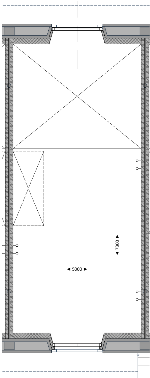
Eerste verdieping
