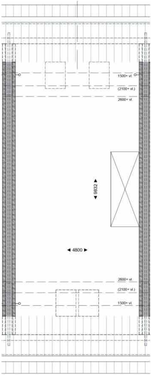
Tweede verdieping
