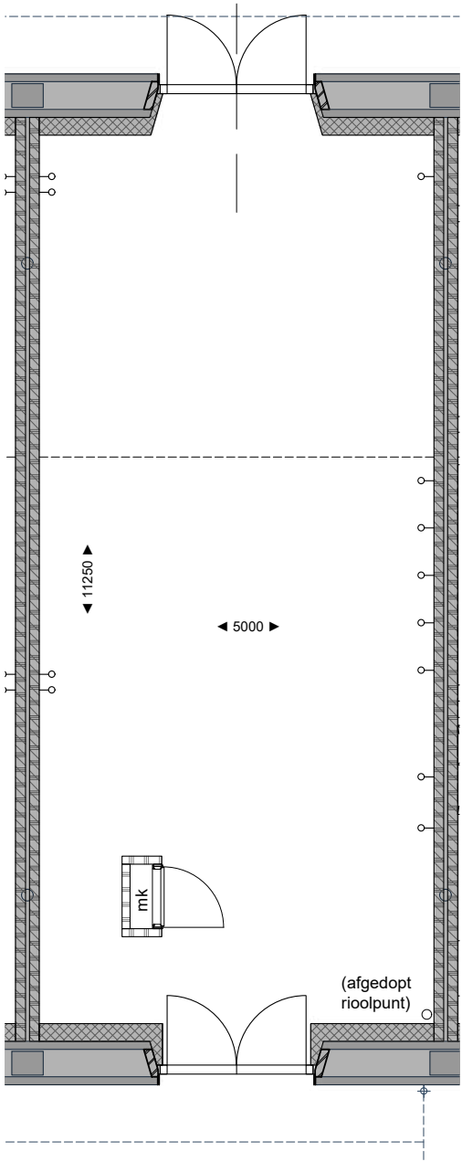
Begane grond
